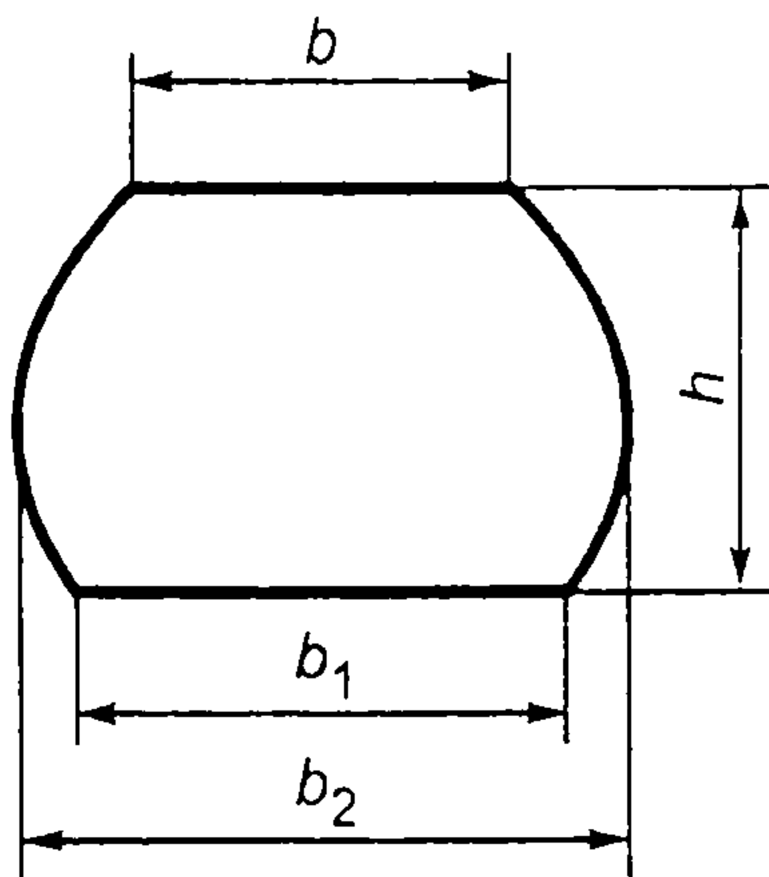
Рисунок 2 – Поперечное сечение бруса вида Б
